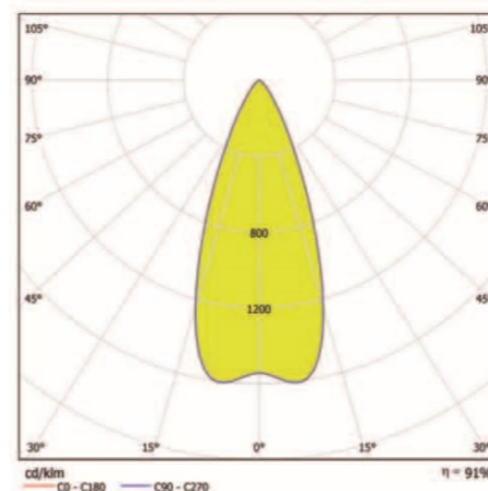
CURVA POLAR 25°
